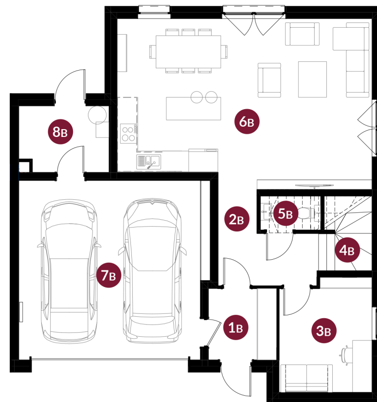
rzut parteru
